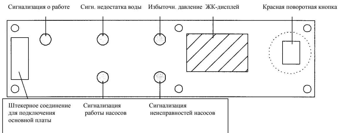
Рис. 5: Плата дисплея
