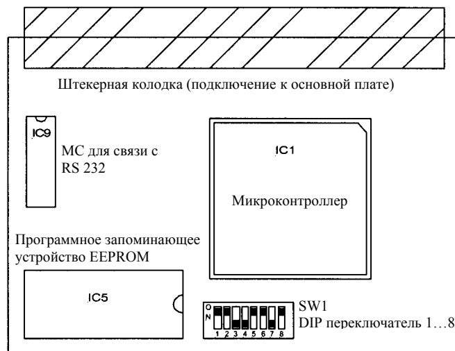
Рис. 4: Плата микроконтроллера
