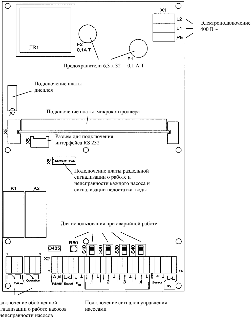
Рис. 3: Основная плата
